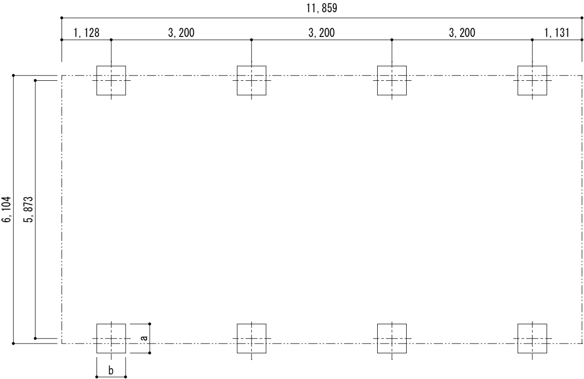
■基礎配置図
